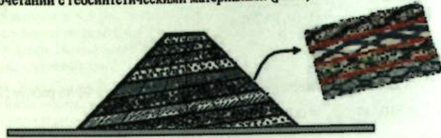
Рисунок 2. Конструкция плотины наклоннослоистого строения.
