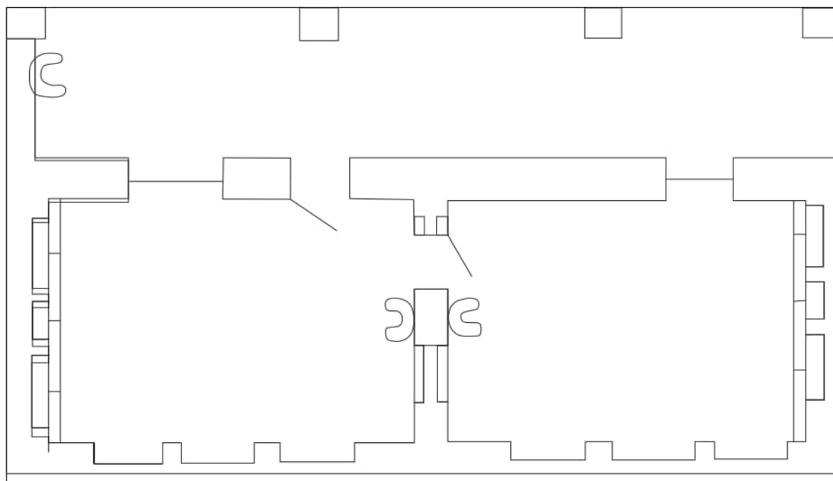
Рис. 1. а) Пеш айван, б) дализ, в) уй; 1-тор, 2- такча, 3- очок, 4- дарча, 5- эшик, 6- устун, 7- мээрап Ошская область, Кара-Суйский район, село Зарбалик. Проект дома Омош ажы
