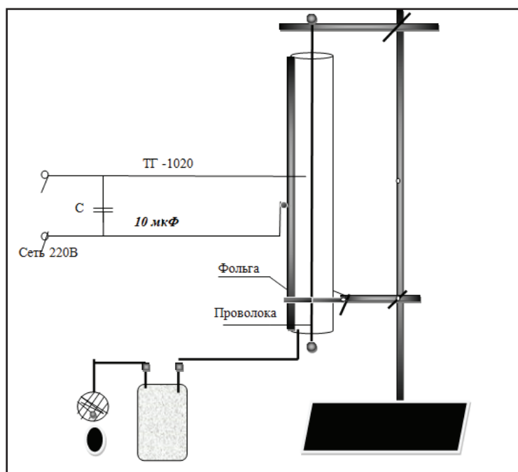
Рис. 2. Коронный разряд
